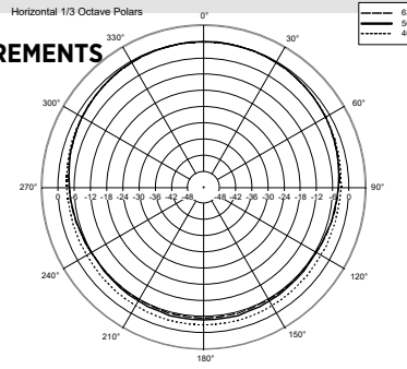
Horizontal 1/3 Octave Polars
